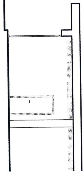
SEZIONE AA STATO DI FATTO 1:100
